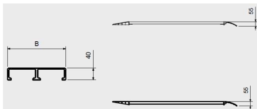
Model met C040-uiteinde (op aanvraag)
