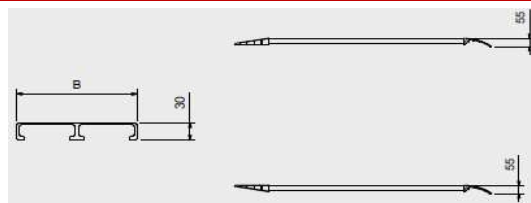
Model met C040-uiteinde (op aanvraag)
