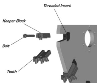
Overzicht onderdelen
